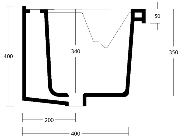
Sezione / Section
