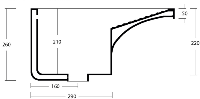
Sezione / Section
