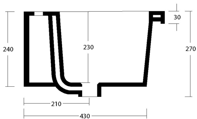
Sezione / Section
